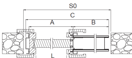
System kasetowy pojedynczy
